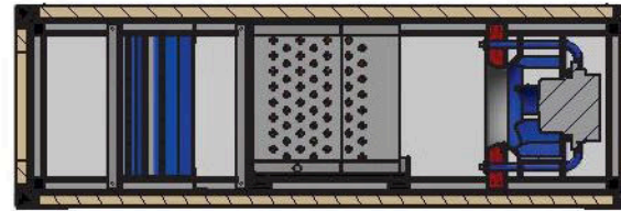
A-A (1 : 12)
